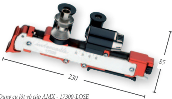
Dụng cụ lột vỏ cáp AMX - 17300-LOSE
